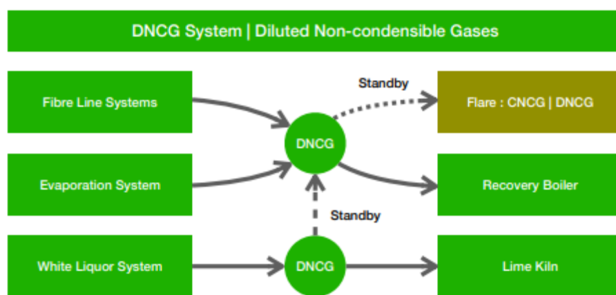
Joonis 1.5. Lihtsustatud lahjade lõhnagaaside (DNCG) käitlus väävelhappe tootmisel [allikas: VKG Fiber tehnoloogilise eelprojekteerimise dokumentatsioon]
