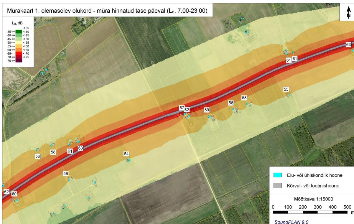
Joonis 3.6. Liikluse müra hinnatud tase päeval (7.00-23.00) olemasolevas liikluskorras
